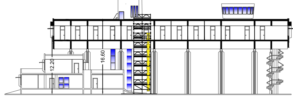
Sezione B - B Scala 1:400
