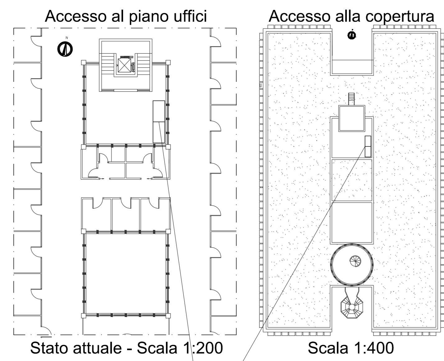
Stato attuale - Scala 1:200
