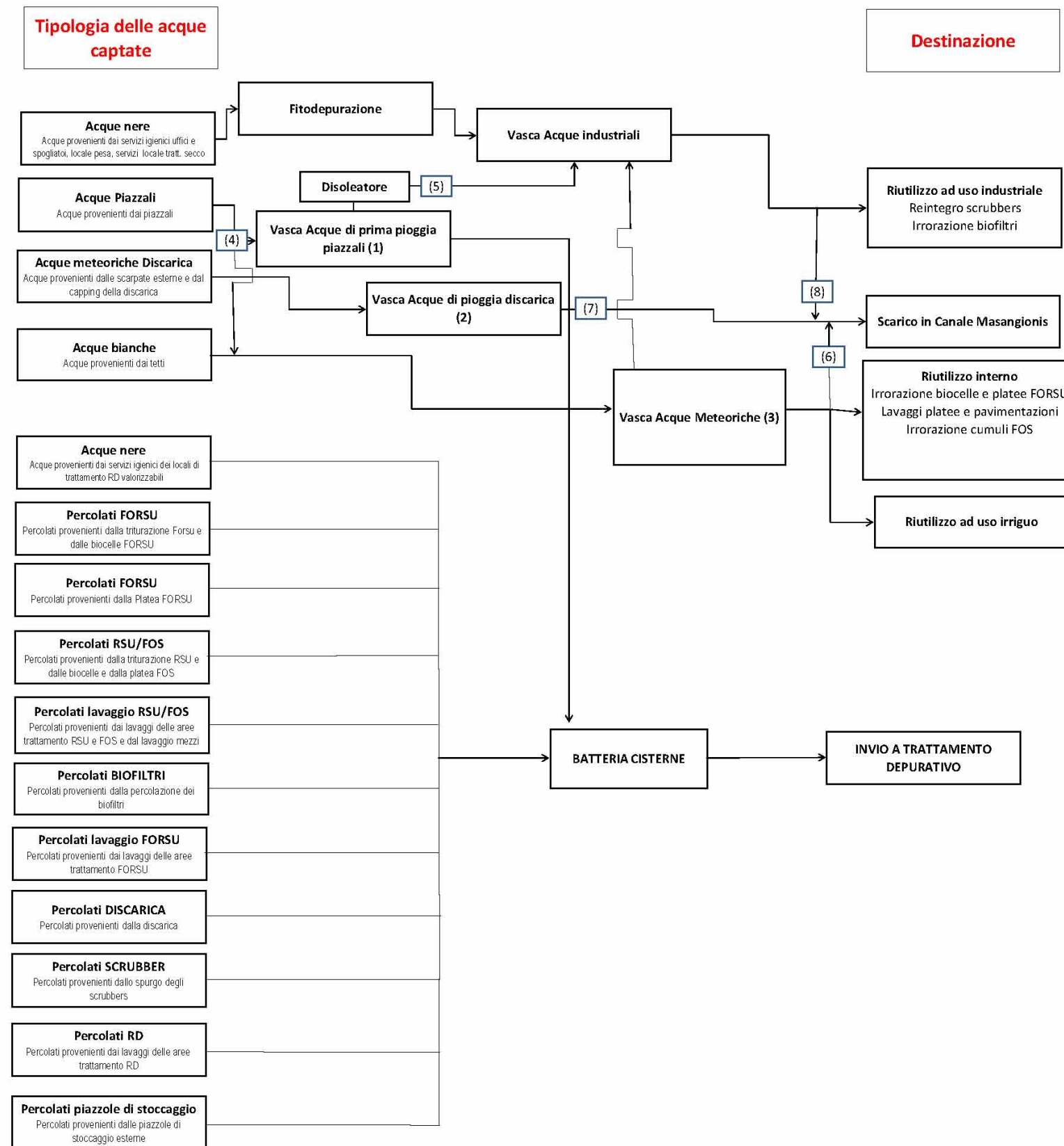
DIAGRAMMA DI FLUSSO DELLE ACQUE
